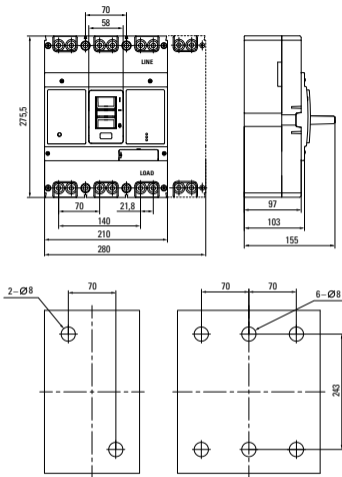
Габаритные размеры ВА-99М 1250 с электронным расцепителем
