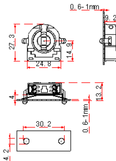
Патрон (ламподержатель) G13 торцевой, встраиваемый в 9,2мм для люминесцентной лампы T8,T12 с пружиной (крепление на цапфы)
