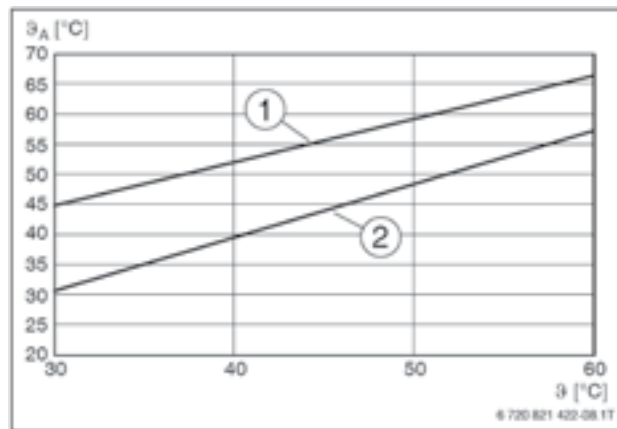
Температура дымовых газов в зависимости от температуры обратной линии котла θ A - Температура дымовых газов θ - Температура обратной линии котла. [1] Полная нагрузка. [2] Частичная нагрузка.
