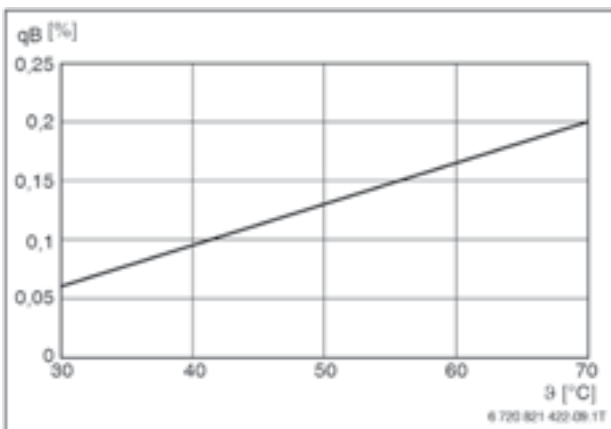
Потери при эксплуатационной готовности в зависимости от температуры обратной линии котла. qB - Потери при эксплуатационной готовности. θ - Температура обратной линии котла.
