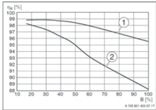
Коэффициент полезного действия в зависимости от нагрузки горелки по высшей теплоте сгорания. ηк - Коэффициент полезного действия B - Нагрузка на горелку в % [1] 40/30 °C [2] 75/60 °C
