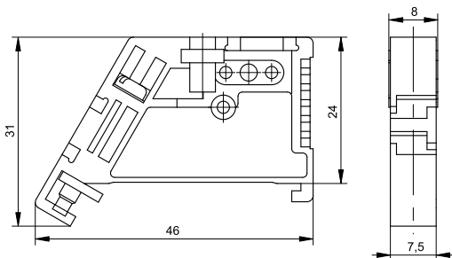
Рисунок 1 – Габаритные размеры ограничителей
