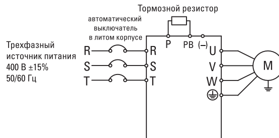
Рисунок 3-3 Стандартное трехфазное подключение 0,75–2,2 кВт
